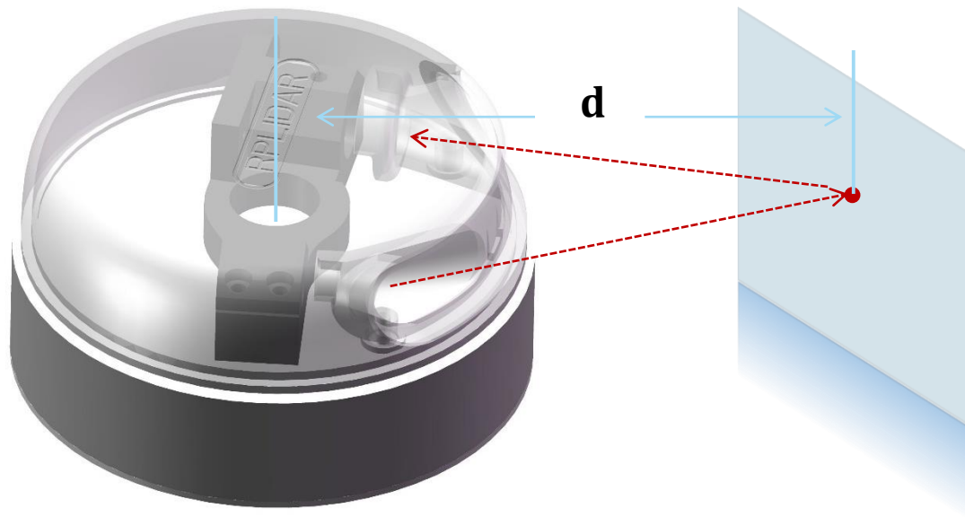
图表 1-2 RPLIDAR A3M1 工作原理示意图
