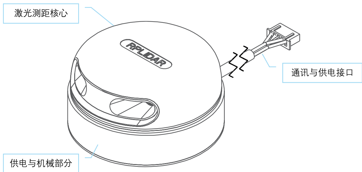
图表 1-1 RPLIDAR A3M1 系统构成示意图
