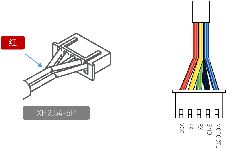
图表 3-1 RPLIDAR A3 模块引脚示意图
