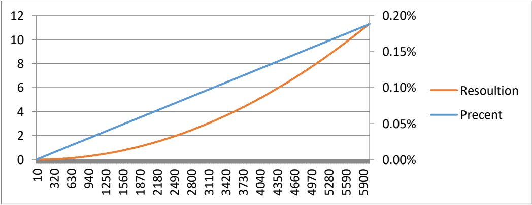
图表 2-2 RPLIDAR A1 测距系统距离分辨率随实际距离变化趋势图
