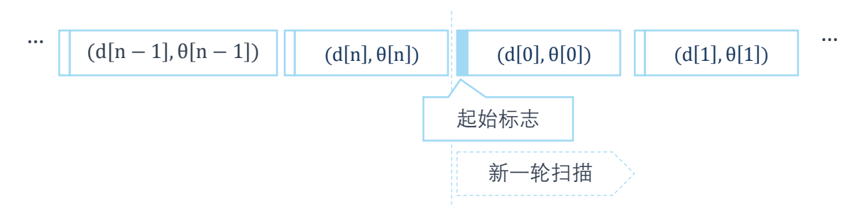
图表 1-4 RPLIDAR A1 采样点的数据信息
