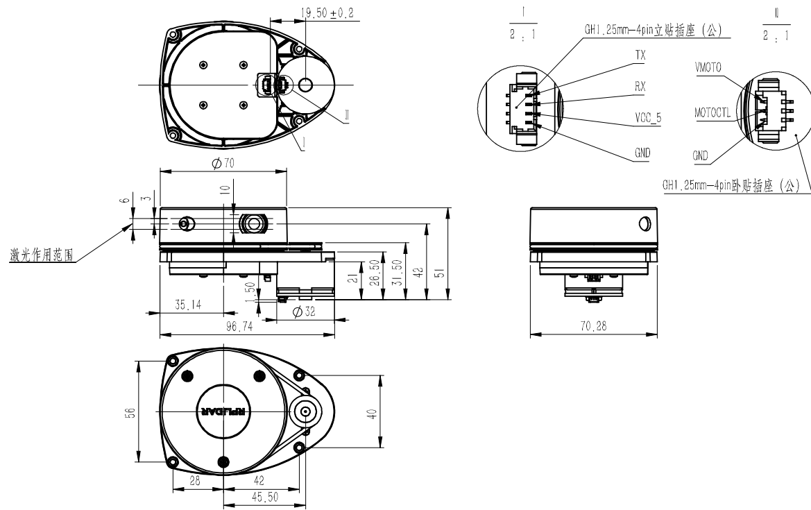
图表 5-2 RPLIDAR A1 机械尺寸图
