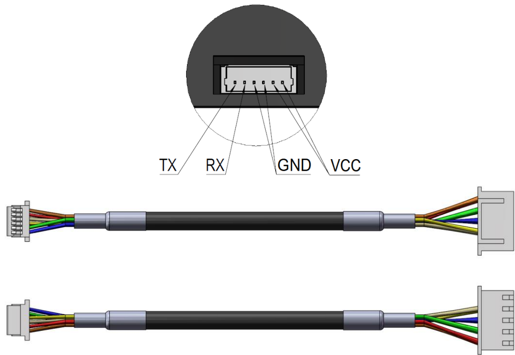
图表 3-1 RPLIDAR S1 接口示意图
